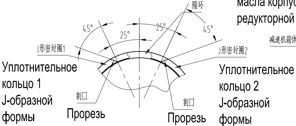
Схема монтажной прорези уплотнительного кольца J-образной формы J型密封圈安装割口示意图
